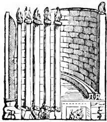
Fig. 560. Præfurnium hypocaust.
